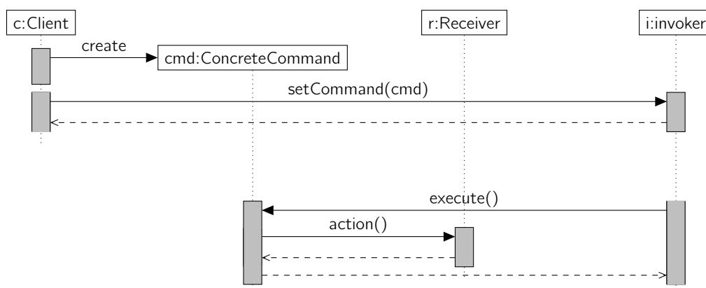
Figure 4 – Diagramme de séquence
