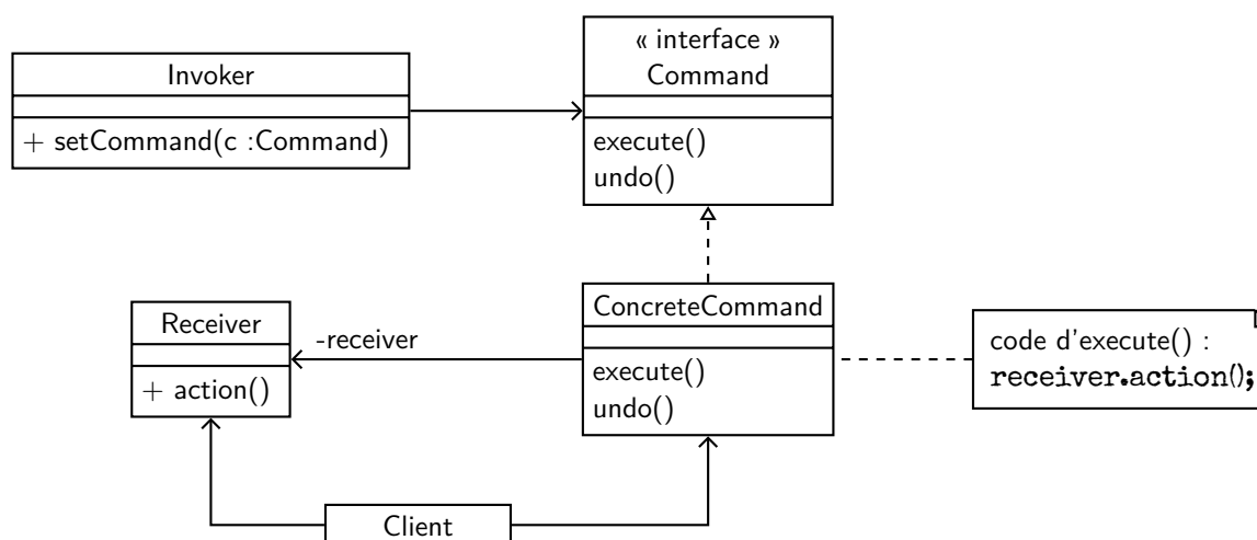
Figure 3 – Patron de conception « Commande »
