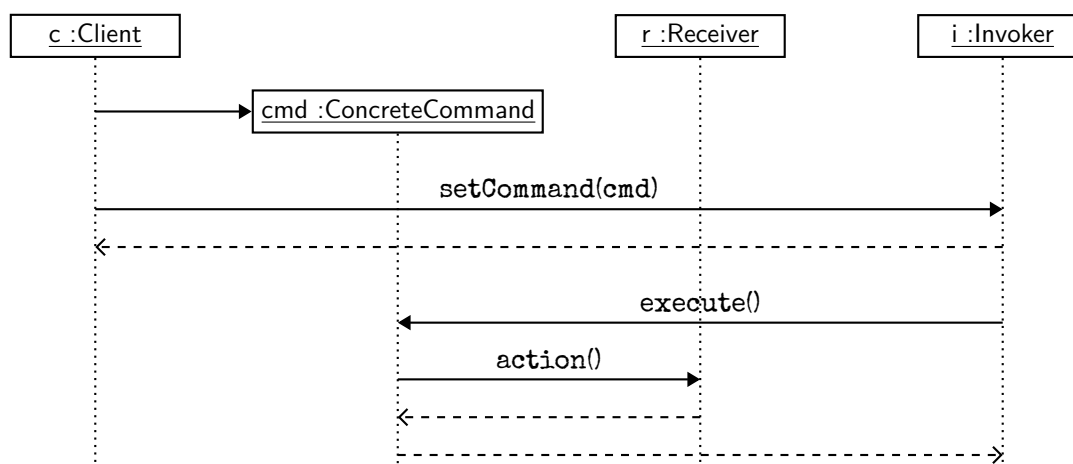
Figure 4 – Diagramme de séquence
